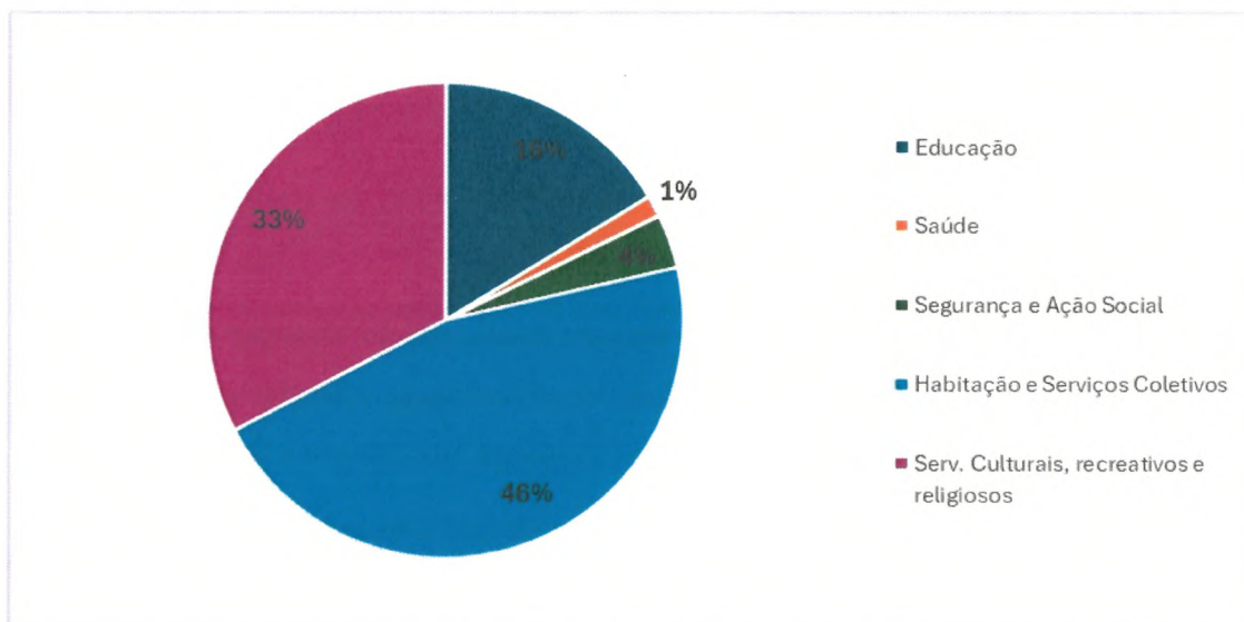
Gráfico 14 - % de Execução das Funções Sociais
